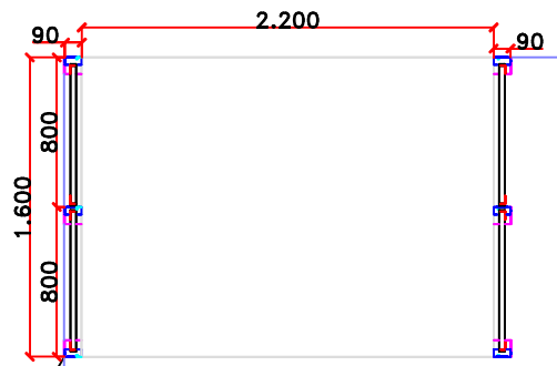
VISTA SUPERIOR
