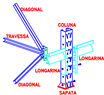
DETALHE ESTRUTURA
