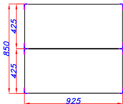
VISTA SUPERIOR 925
